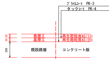
施工要領図
